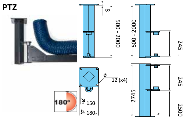
Fijaciones de techo y de suelo para el extractor Fumex PR, en las longitudes de 5 y 7 m. Giro de 180°.
