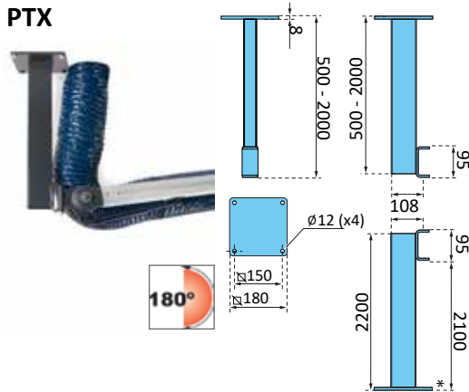
Fijaciones de techo y suelo para el extractor Fumex PR, en las longitudes 1,5, 2, 3 y 4 m. Giro de 180°.
